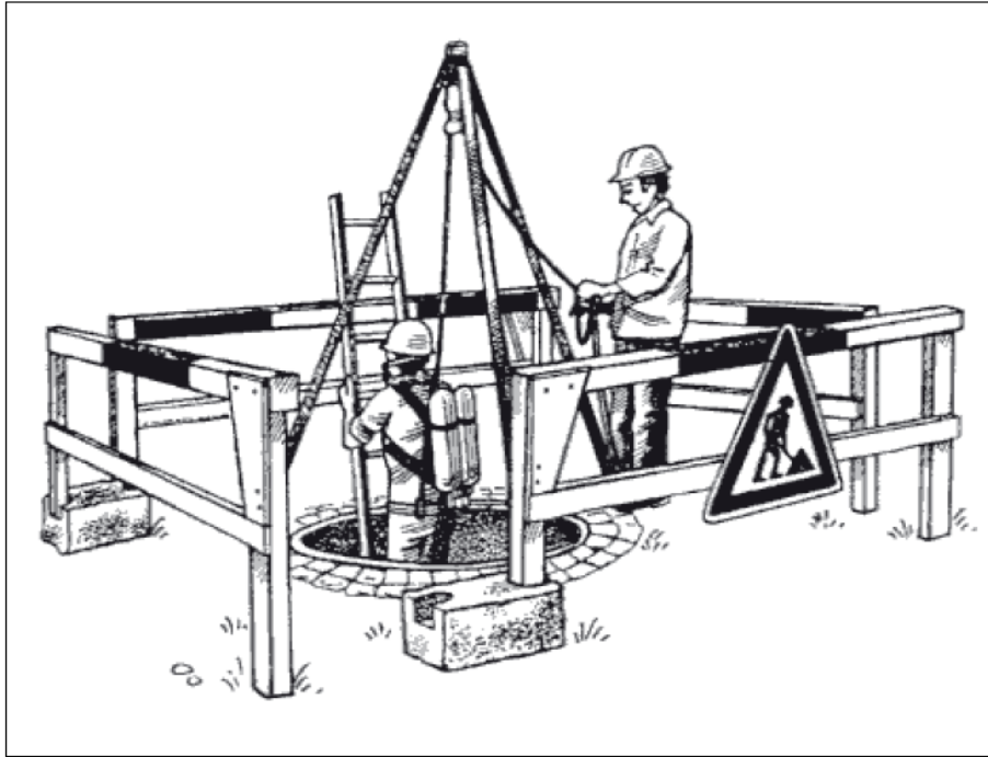
شکل ۳-۴ - ایمنی در ورود به فضاهاى محبوس
