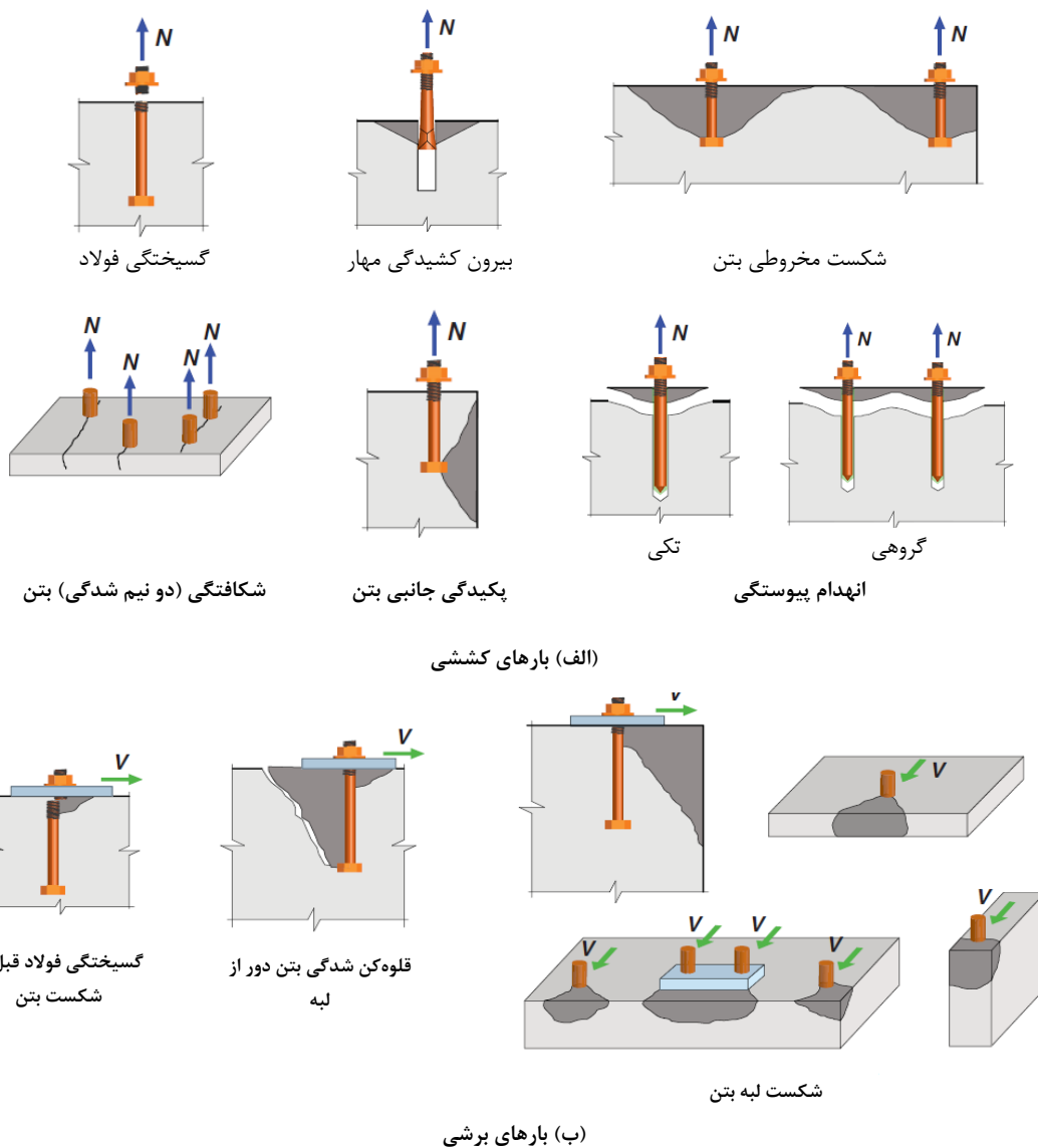
شکل ۱۸-۳ انواع حالات شکست مهارها در کشش و برش
