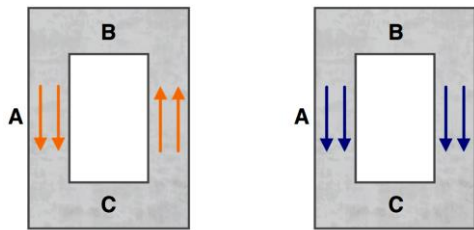
تنش‌های برشی ناشی از برش الف - مقطع توخالی (جعبه‌ای)
