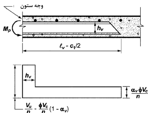
شکل ۷-۸ برش ایده‌آل در کلاhek برشی
