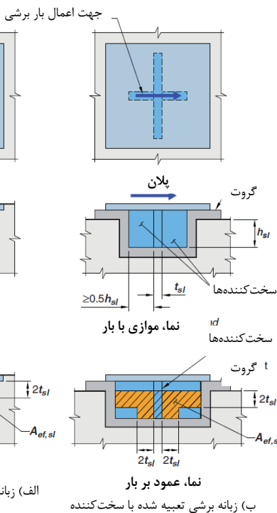
ب) زبانه برشی تعبیه شده با سخت کننده
